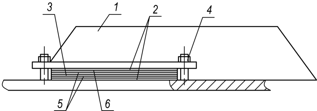
Рисунок 17 – Будова діафрагми
