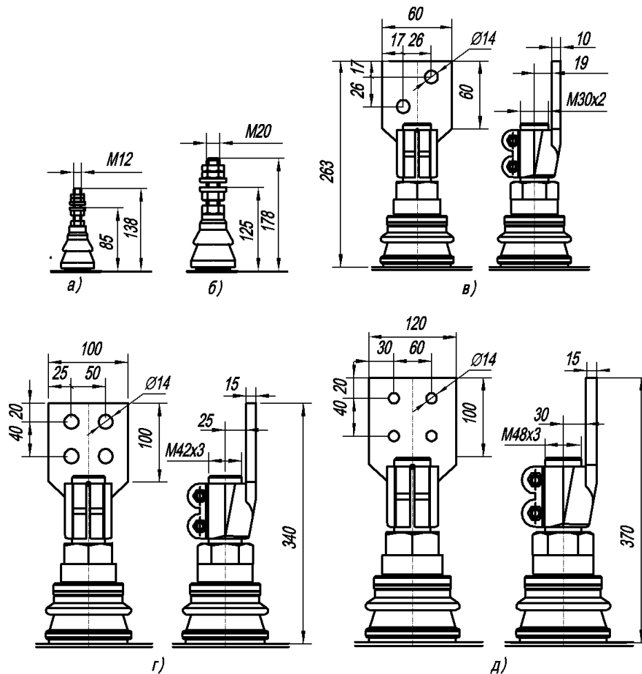
Рисунок 1 – Загальний вид вводів
