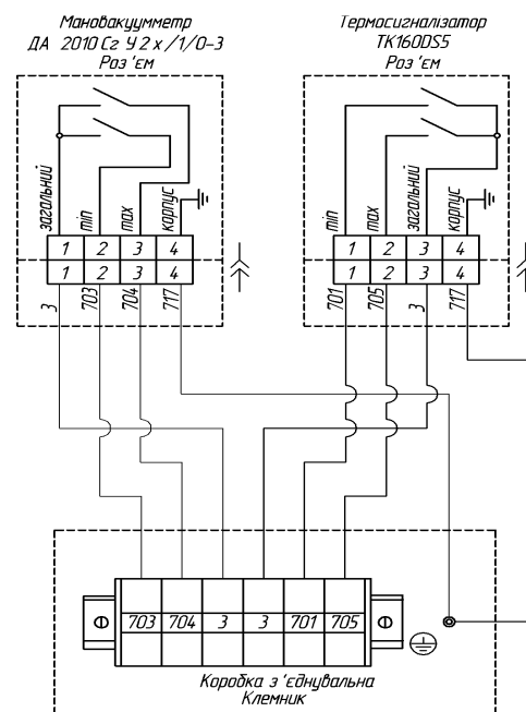
Рисунок 4 – Схема підключення контрольних і захисних приладів трансформатора ТМЗ
