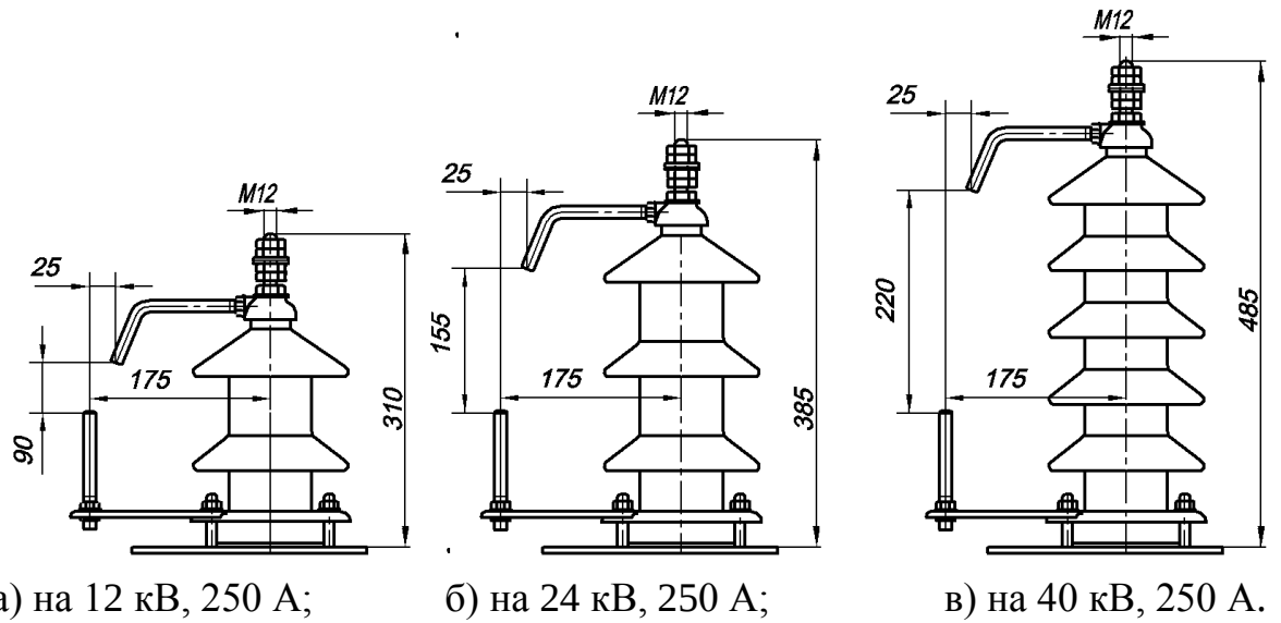
Рисунок 1 – Загальний вид вводів
